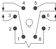
3TX7127 (DPDT)
