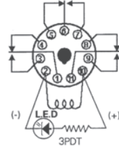
3TX7115
