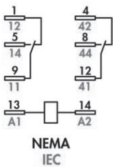
3TX7114
