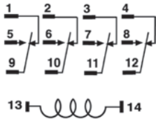
3TX7127
