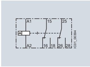
3RP2505-.B (D) Flashing, symmetrical, starting with interval
