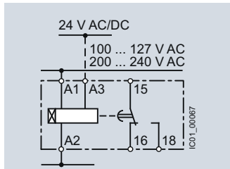
7PV151.-1AQ30, 7PV151.-1AP30 ON-delay
