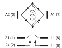
3TX7131 (DPST-NO) (AC)
